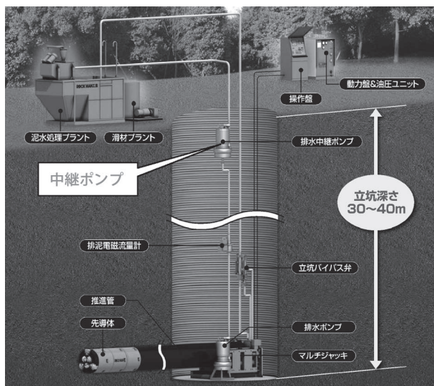
図-8 施工模式図
