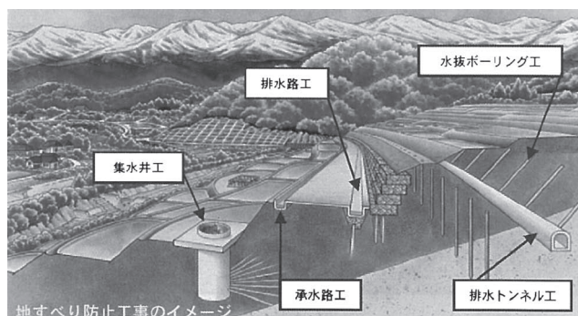
図－3 地すべり対策工事 出典：直轄地すべり対策事業庄内あさひ（農林水産省資料）より
