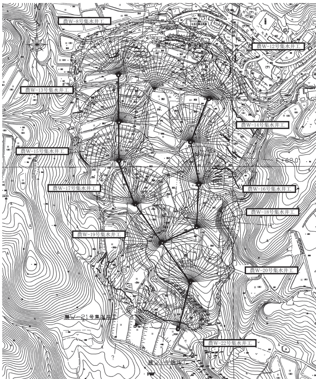
図－４ 地すべり対策工事の概要図
