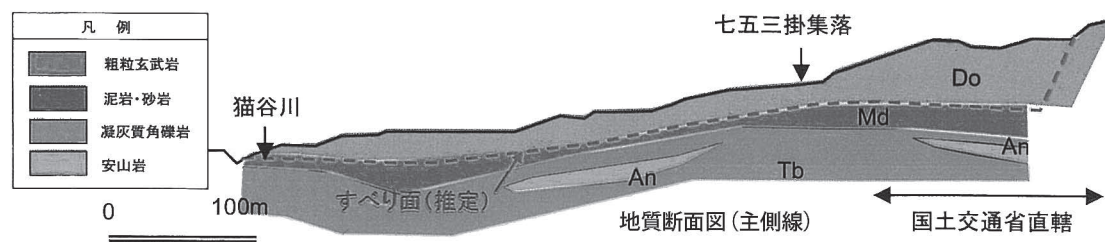
図－２ 七五三掛地区の地質構成 出典：「七五三掛地区地すべりへの対応」国土交通省東北地方整備局新庄河川事務所資料より
